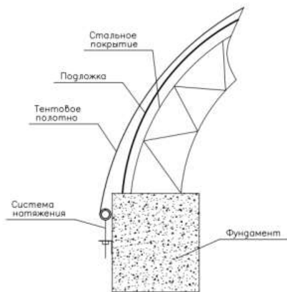
Схема укрытия ангара
